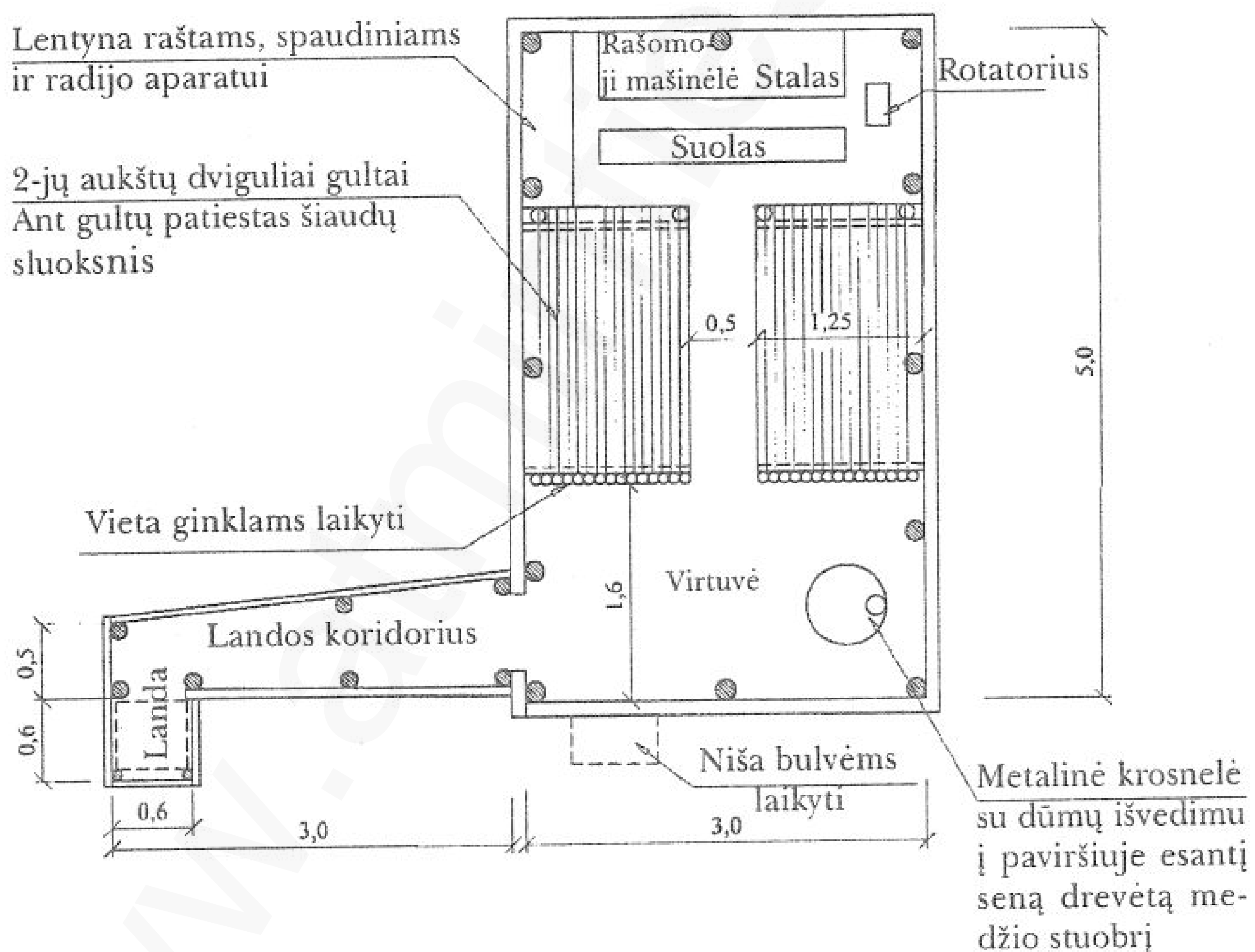
Brėžinys Nr. 2
